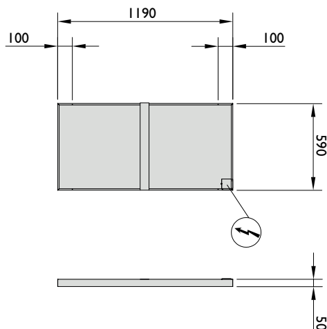
CEILFIT 1200E
