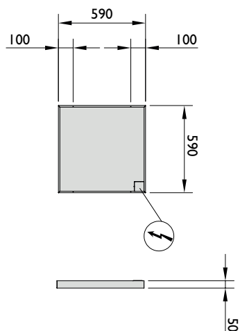
CEILFIT 600E
